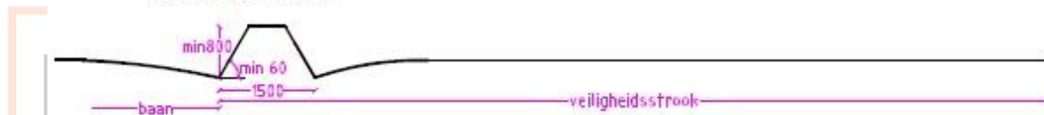
TEKENING 7.1.2 B
