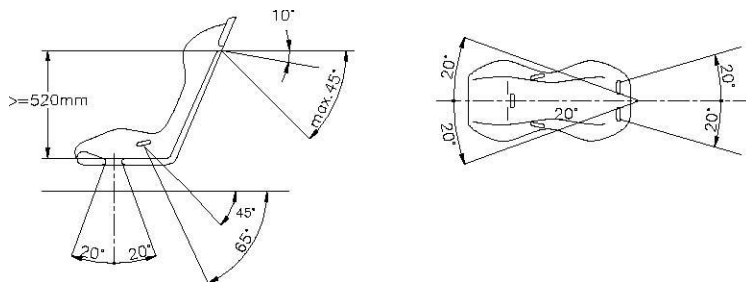
Tekening 253-61
