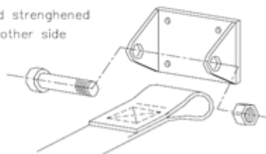
Tekening 253-63
