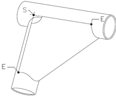
Tekening 253-34
