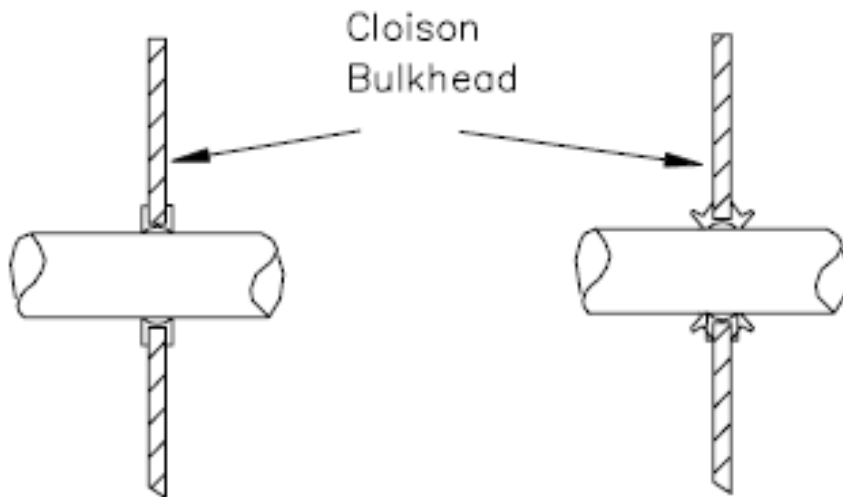
Tekening 253-60
