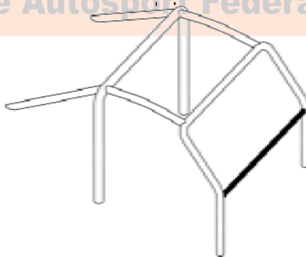
Tekenning 253-29
