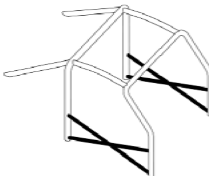
Tekenning 253-9
