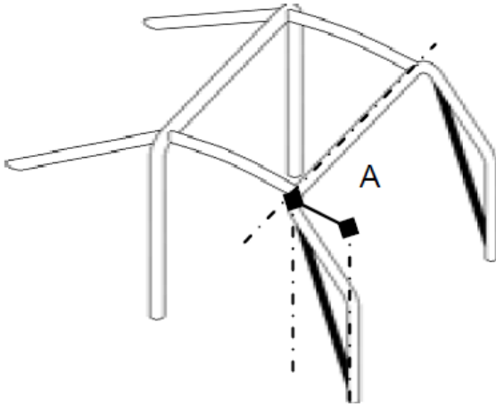
Tekening 253-15
