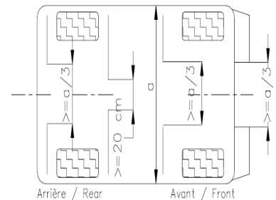
Tekening 253-14
