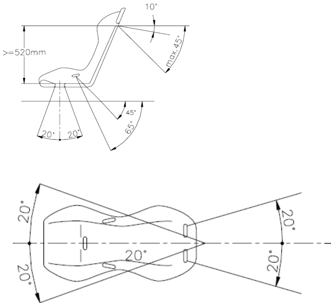
Tekening 253-61
