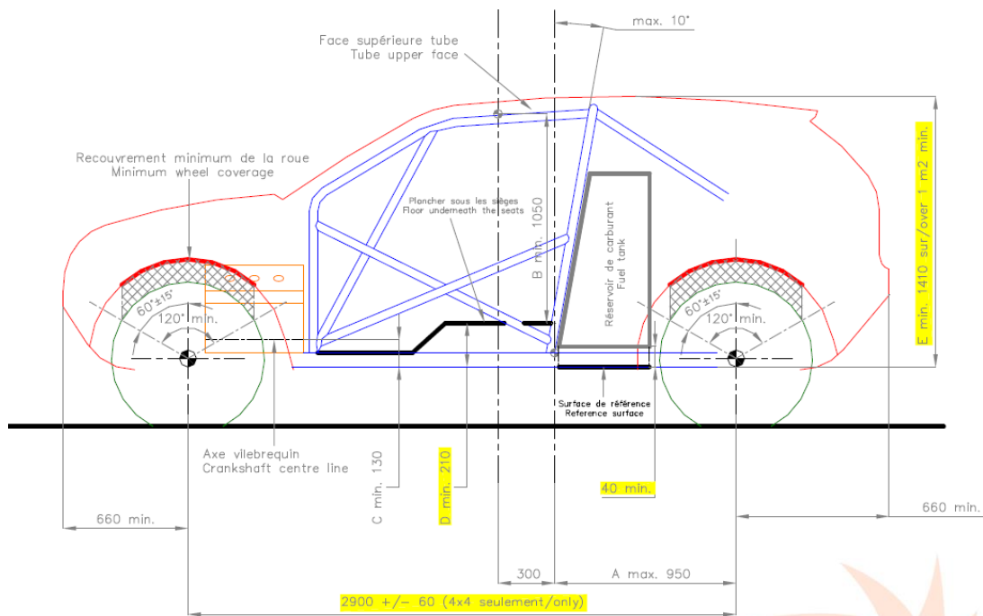
Tekening 285-1
