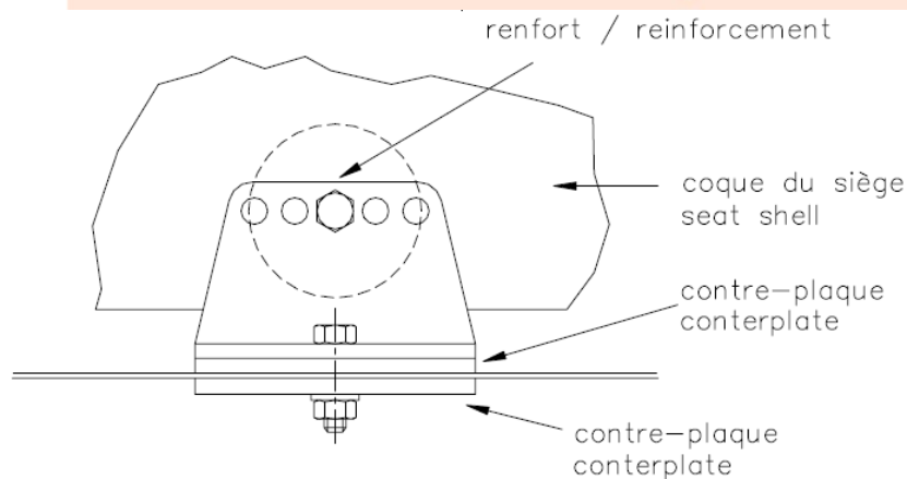
Tekening 253-65
