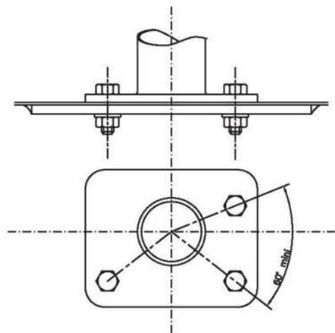
Dessin/Drawing 253-50
