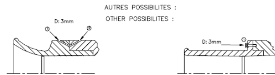
Tekening 254-4
